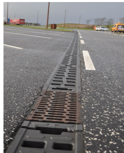
Inspektionsenhed, med mulighed for rense renden. Denne er med låsbar riste i støbejern.
