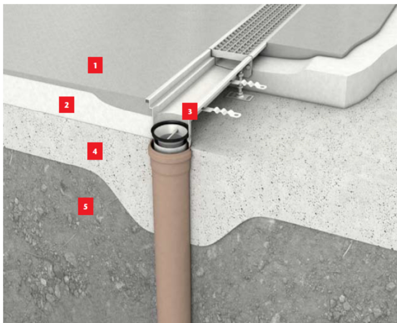
Eksempel på installation: Modular 125 direkte tilsluttet afløbsrør Se øvrige henvisninger i ACO Produktkatalog ACO Modular render
